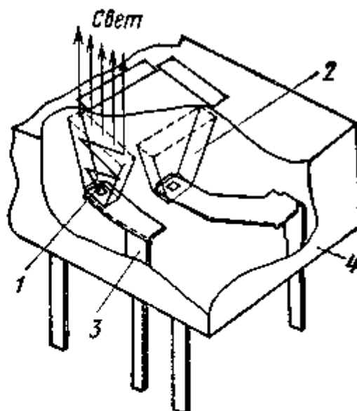
Рис 36 Индикатор с увеличением изображения: 1 — излучающий кристалл; 2 — конический псевдосветовод с металлизированными стенками; 3 — металлическое основание-рамка, 4 — пластмассовый корпус
